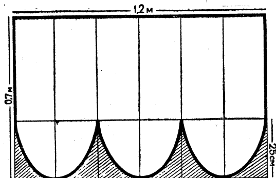
Выкройка мешка для сачка.
